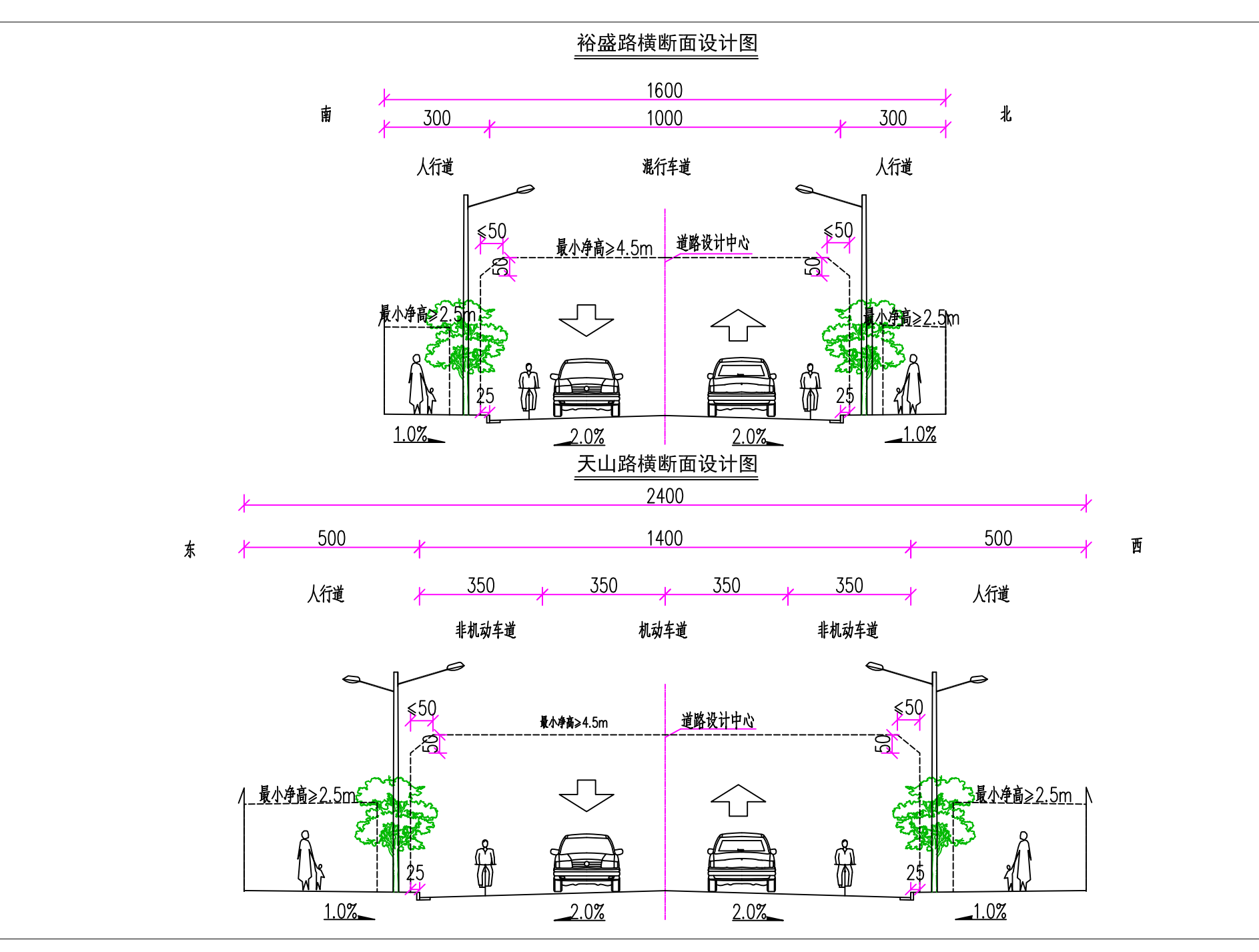
道路标准横断面
